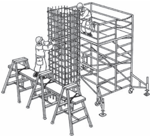
脚立単体では足場に該当しないが、足場板を掛け渡すと足場に該当
